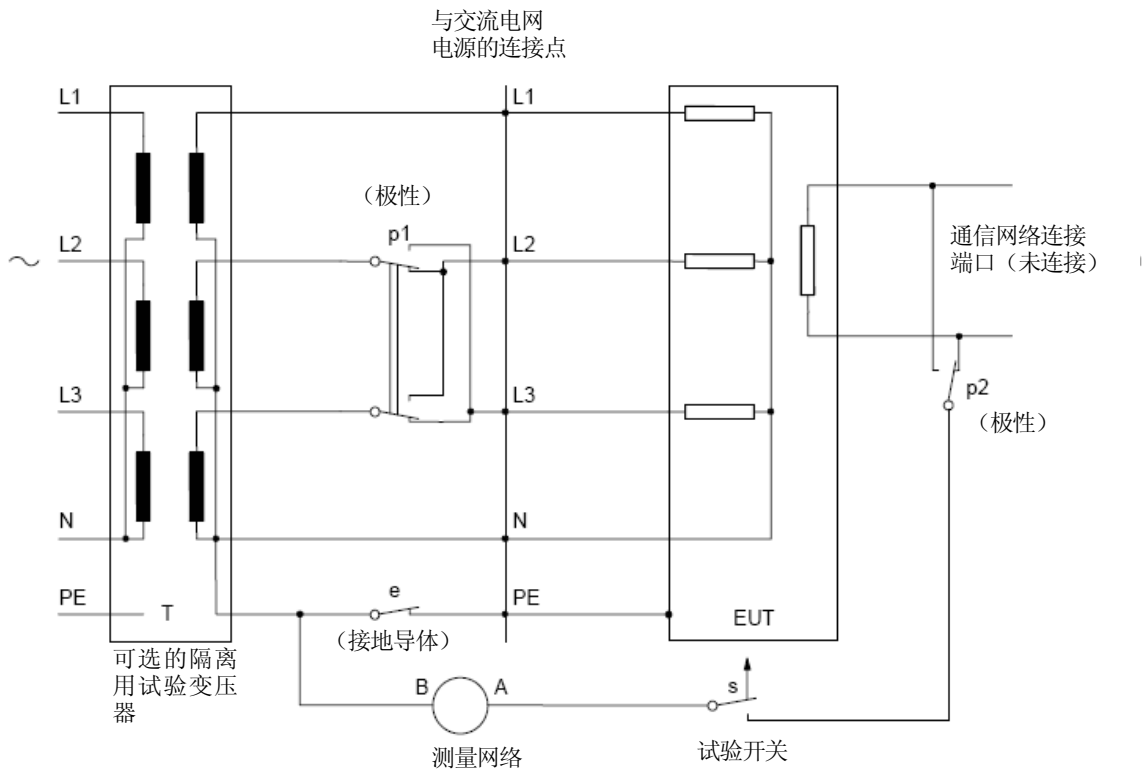
图 5B 接到星形 TN 或 TT 配电系统的三相设备接触电流试验电路
