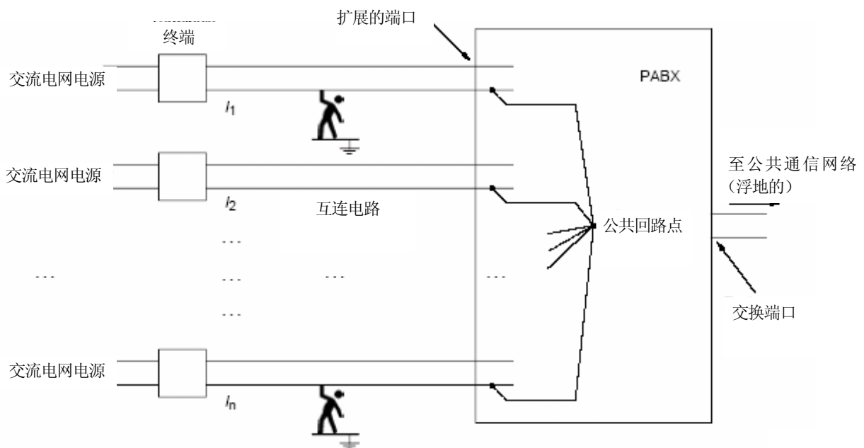
图 W. 3 接触电流在 PABX 内的汇合
