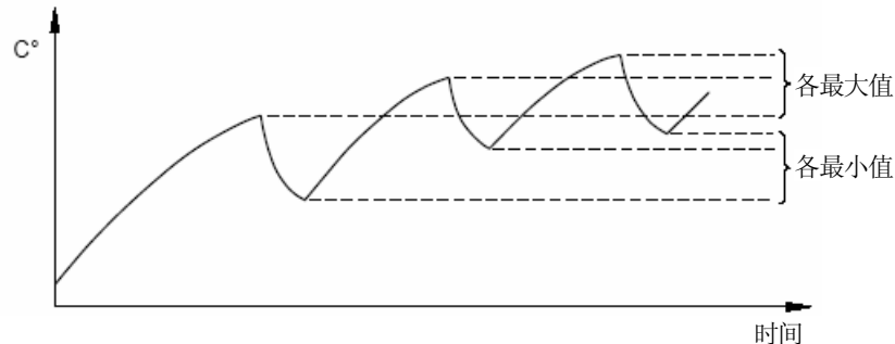
图 C.1 算术平均温度值的确定
