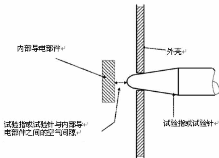
图 2C 试验探头
