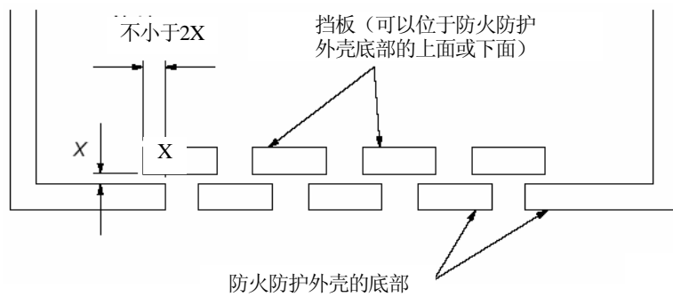
图 4F 挡板结构
