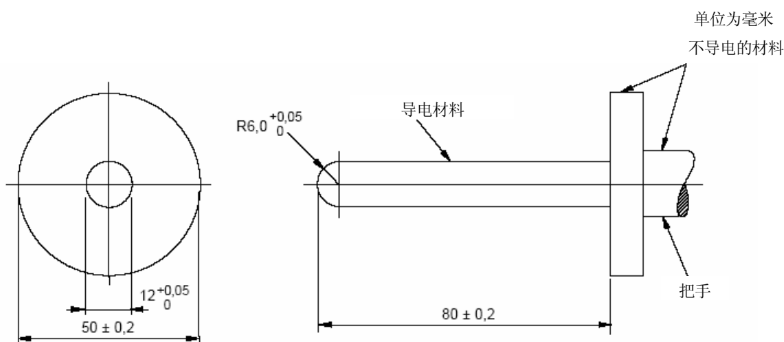
图 2C 试验探头
